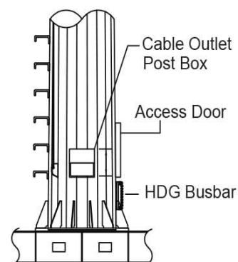
Access Door
